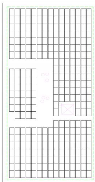
Legplan zonnepanelen
