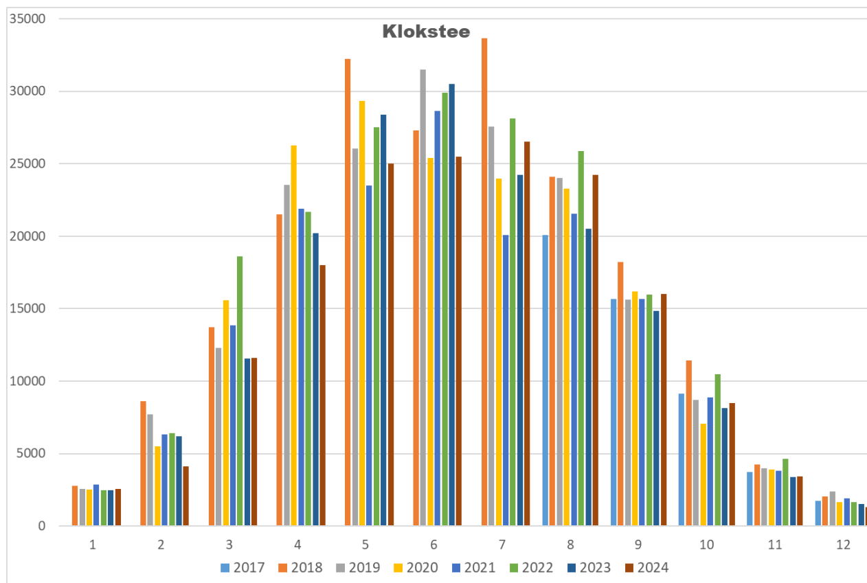
(Fudura) Opbrengst "de Klokstee"(in kWh)
